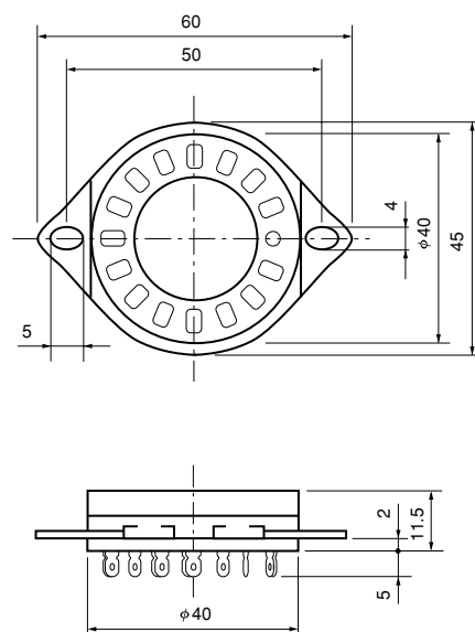
Socket (E678-15B)
