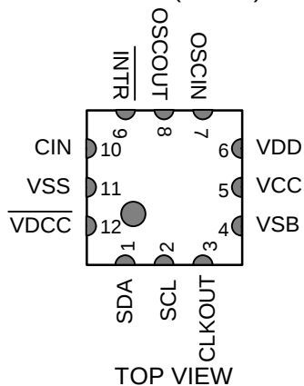
R2051Kxx(FFP12)
