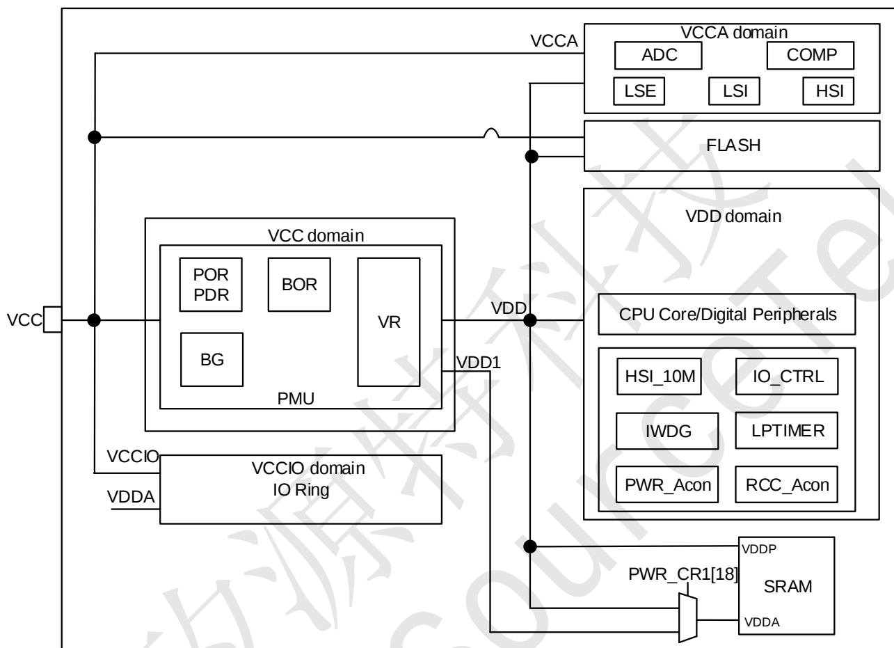
图 2-2 电源框图
