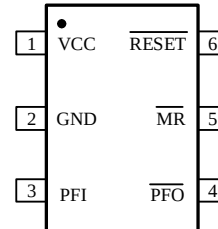
SOT23-6
