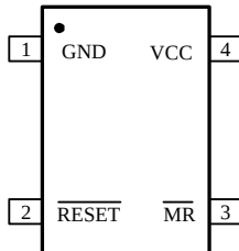
SOT143
