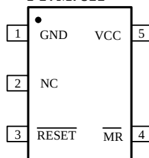
SOT23-5
