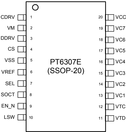
图 3. 管脚定义图
