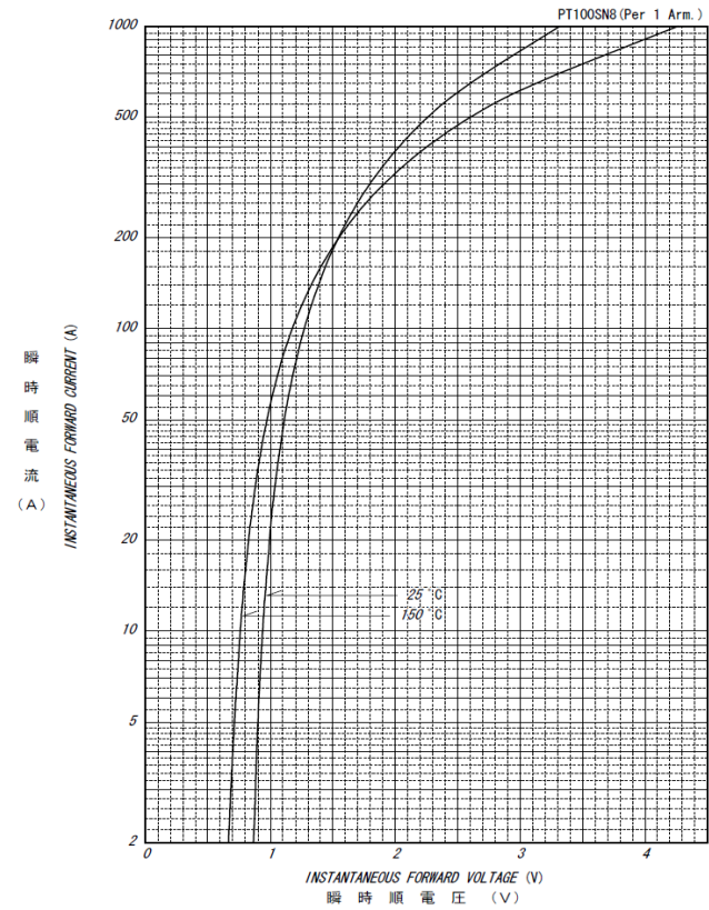
順電圧特性 FORWARD CURRENT VS. VOLTAGE
