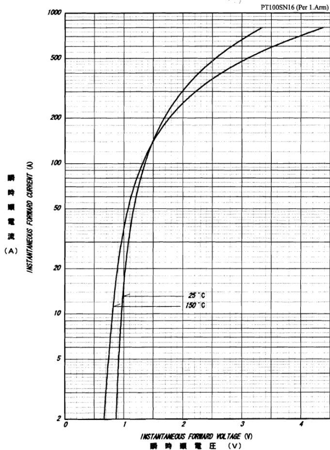
順電圧特性 FORWARD CURRENT VS. VOLTAGE
