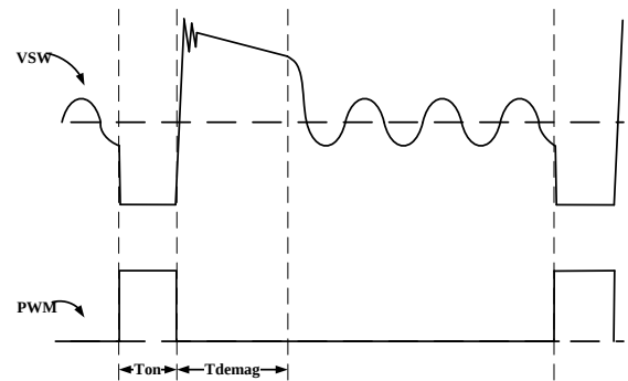
图5.准谐振模式
