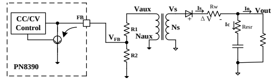
图4.线补电流
