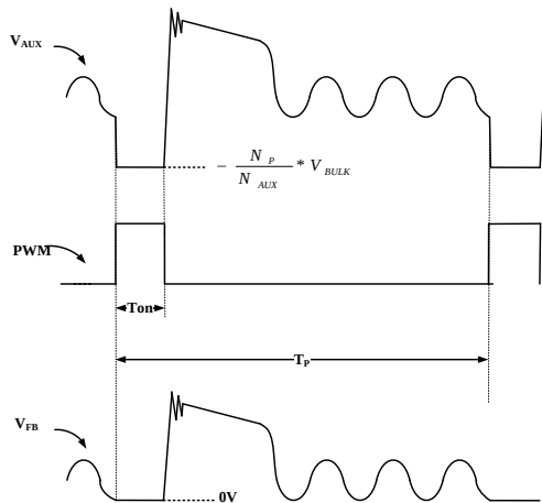
图3.输入电压检测波形
