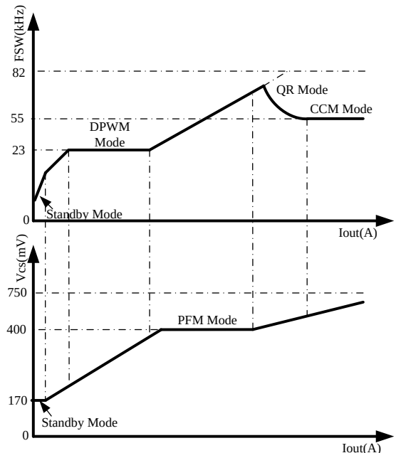
图1.工作频率、Vcs和负载关系
