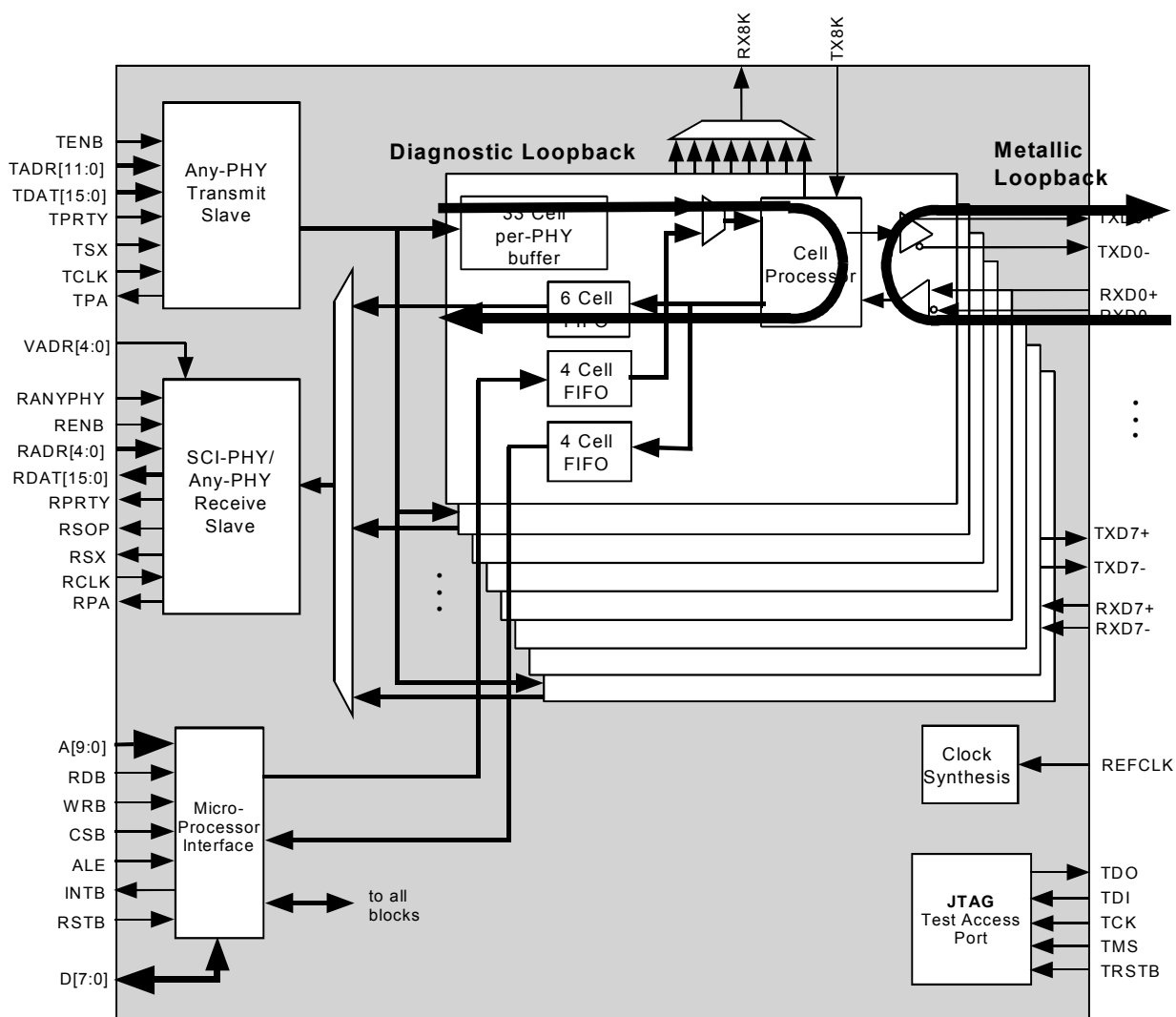
Fig. 5 Loopbacks
