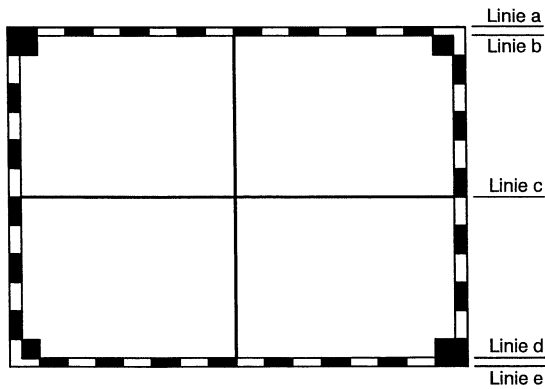
Fig. 4 Mittenkreuz, 625 / 525 Zeilen, Bildformat 4:3
