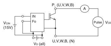
Fig. 5 I_{CES} Test
