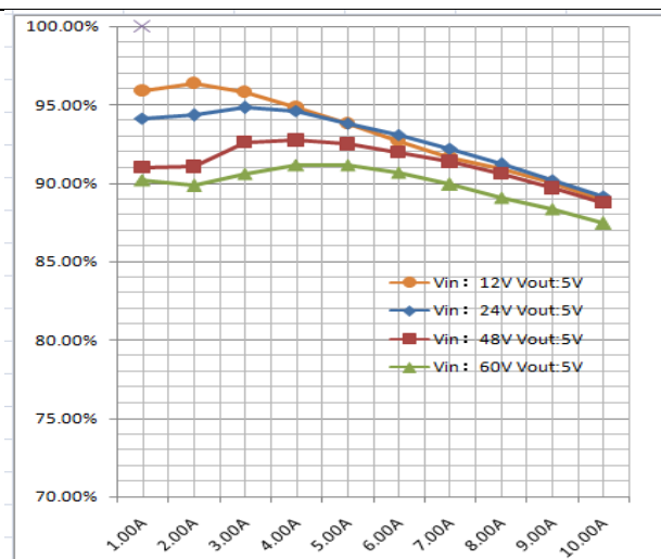
Fig. 4 效率曲线
