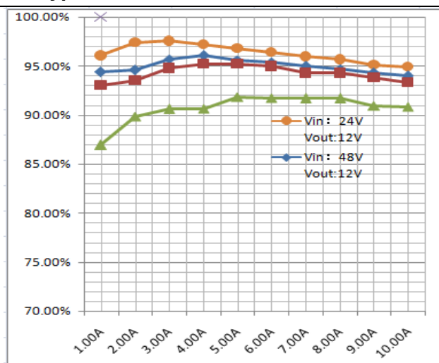
Fig. 3 效率曲线
