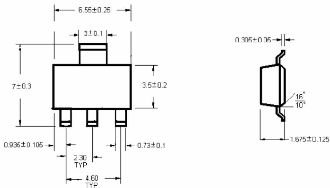
SOT-223 Unit:mm
