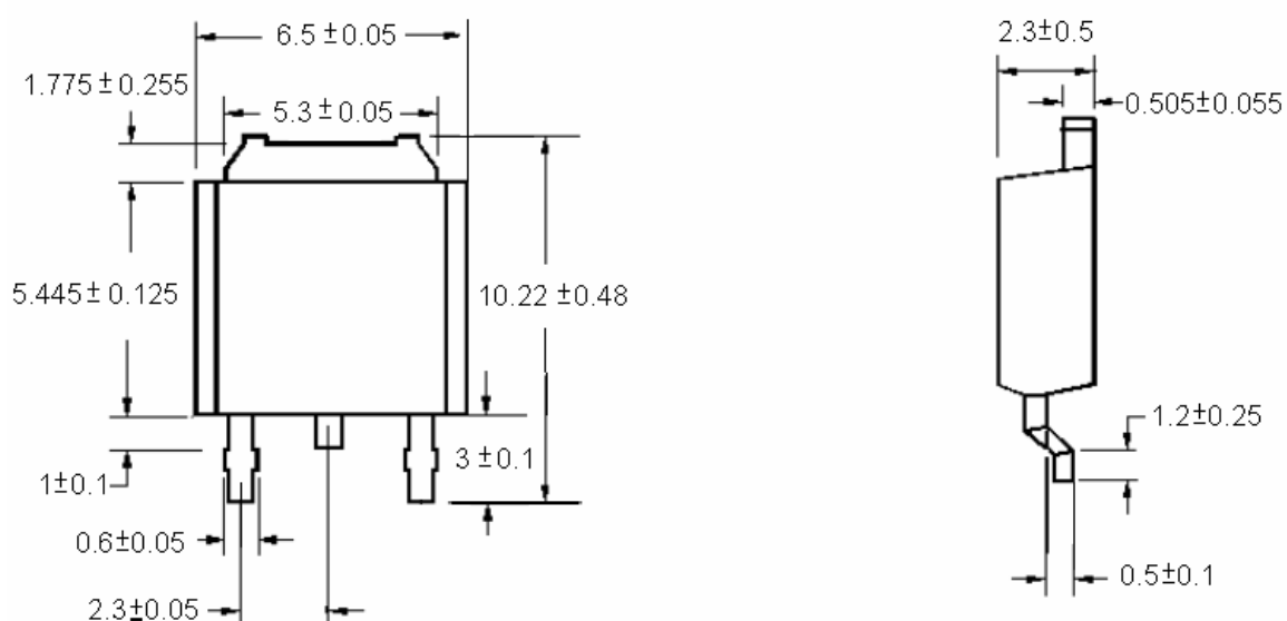
TO-252 Unit:mm
