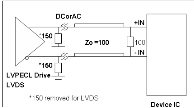
LVPECL/ LVDS Input
