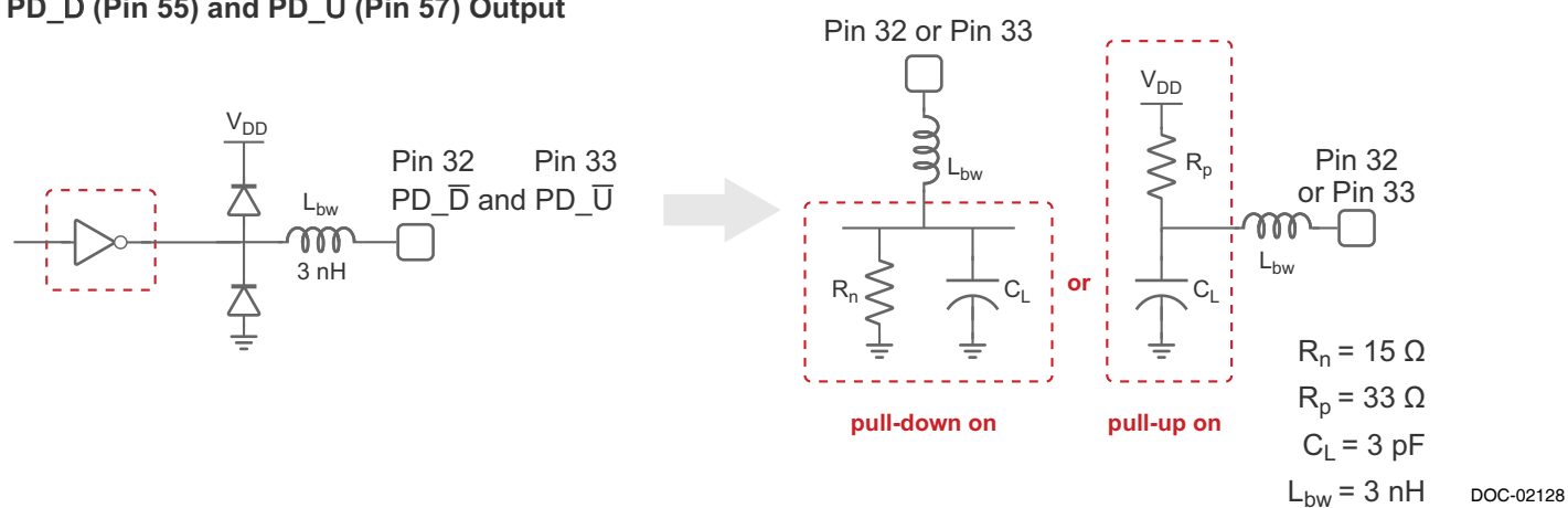
PD_D (Pin 55) and PD_U (Pin 57) Output
