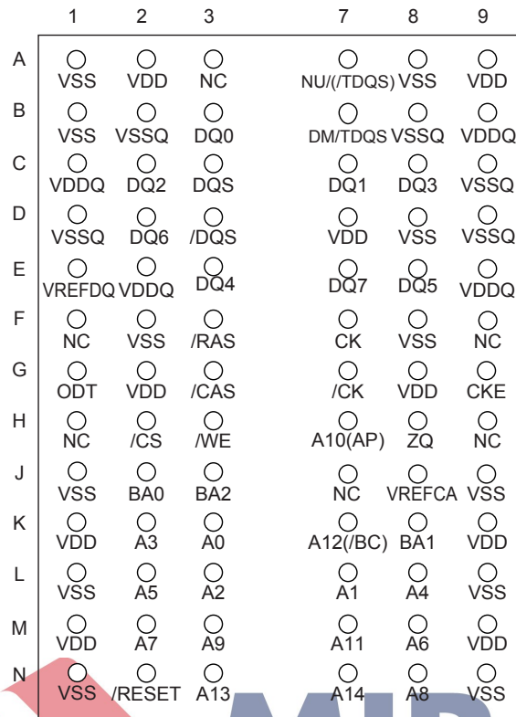
78-ball FBGA
