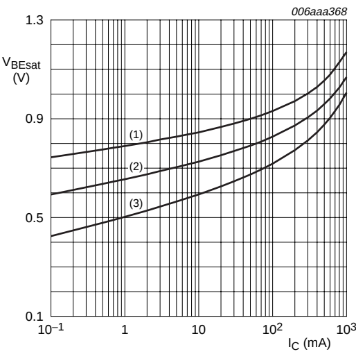
I_C/I_B = 20 (1) T_{amb} = -55^\circ C (2) T_{amb} = 25^\circ C (3) T_{amb} = 100^\circ C
