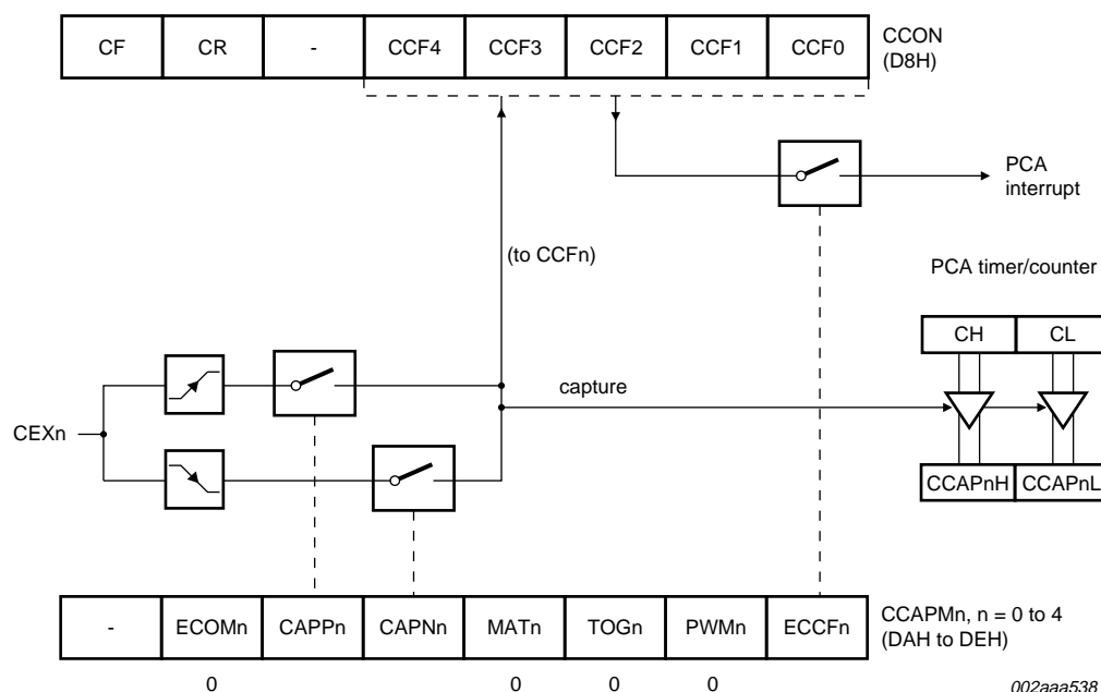
Fig 22. PCA capture mode
