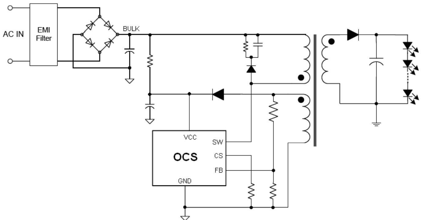
图一， OCP8154 典型应用电路
