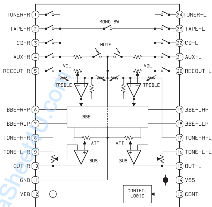
IC, M61503FP
