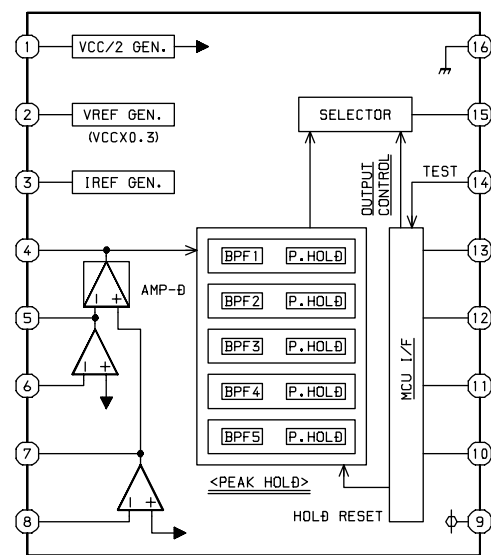
IC, M61506FP
