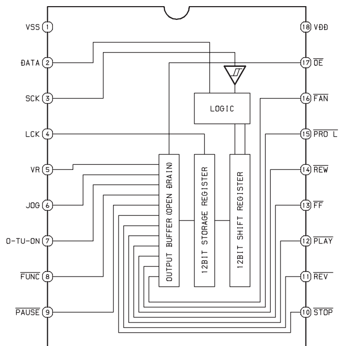
IC, BU2092F
