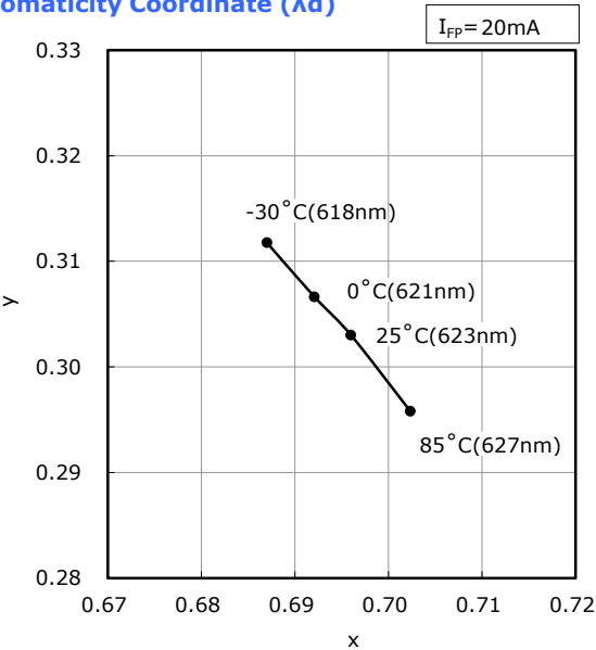
周囲温度-色度(主波長)特性 Ambient Temperature vs Chromaticity Coordinate ( \lambda_d )
