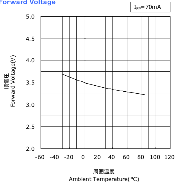
周囲温度-順電圧特性
