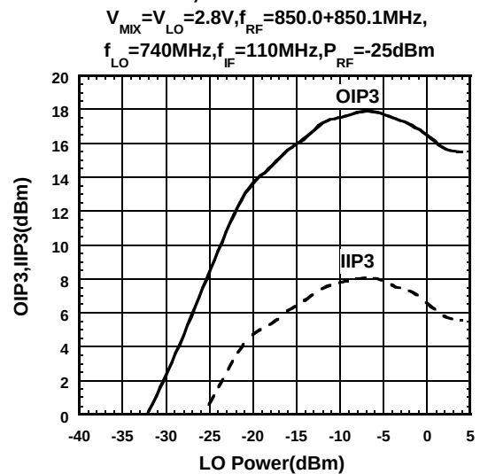
OIP3, IIP3 vs. LO Power
