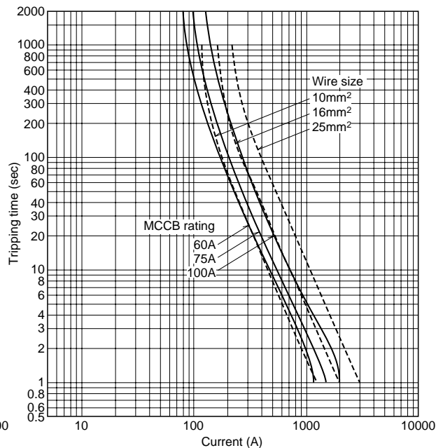
b) 100A-fream MCCB
