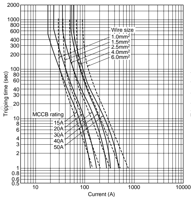
a) 50A-fream MCCB
