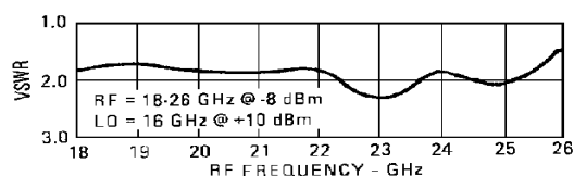
R-Port VSWR
