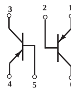
PNP+PNP
