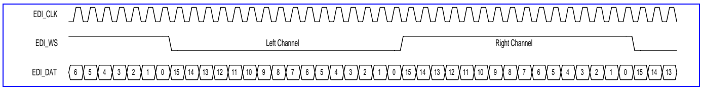
Figure 59 EDI Format 1: EIAJ (FMT = 0).
