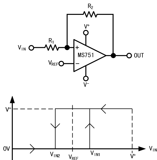
图2 非反向迟滞比较器电路
