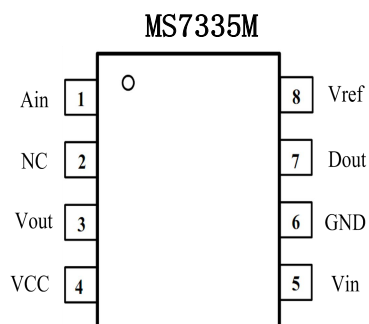
图 1. MSOP-8 外形图
