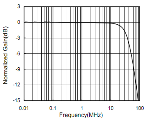
图 2. 频率响应
