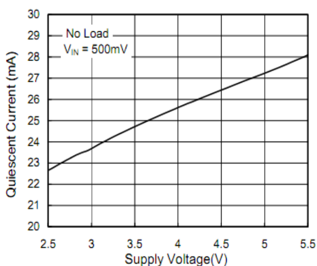
图 9. 工作电流与电源电压的关系
