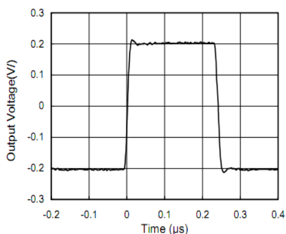
图 4. 小信号阶跃响应
