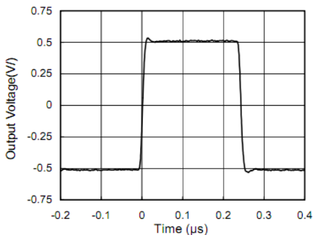
图 3. 大信号阶跃响应
