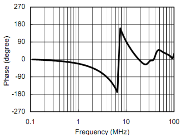
图 2. 相位与频率的关系
