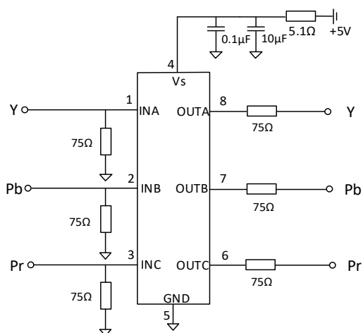
图 13. 直流耦合应用原理图
