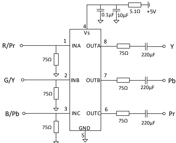
图 14. 直流耦合输入和交流耦合输出应用原理图
