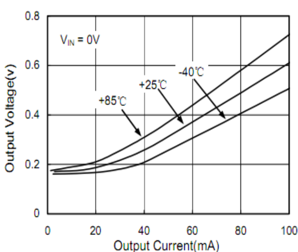
图 12. 负隔离输出电压摆幅与输出电流的关系
