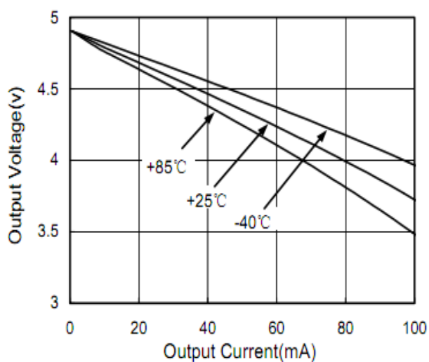
图 11. 正隔离输出电压幅度与输出电流的关系
