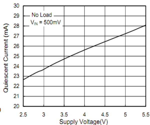
图 8. 静态电流与电源电压的关系
