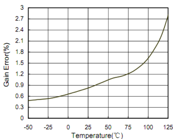
图 10. 增益误差与温度的关系
