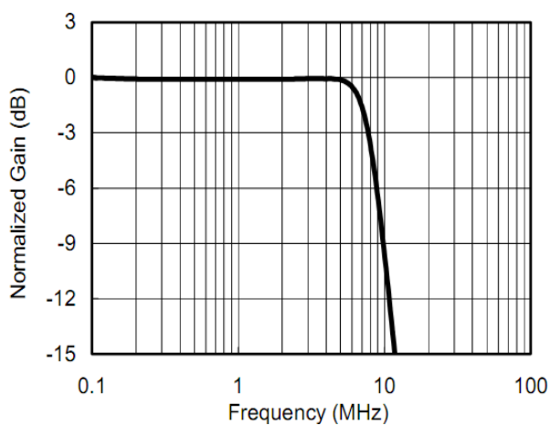
图 1. 频率响应
