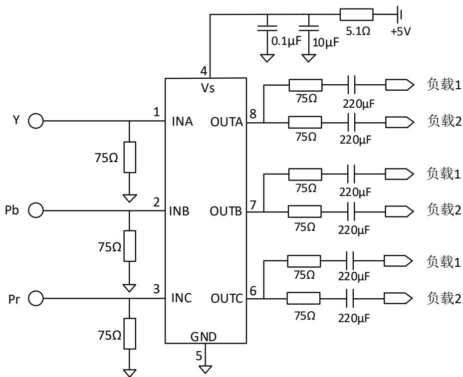
图 15. 机顶盒中直流耦合电路原理图
