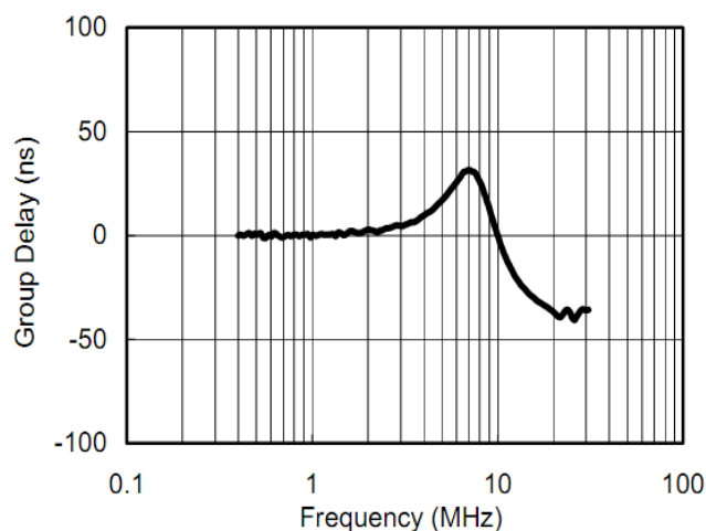
图 7. 群延时与频率的关系
