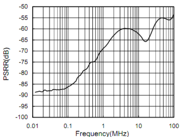
图 5. 电源抑制比与频率的关系 (有旁路电容)
