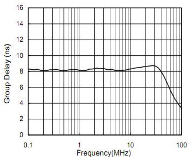
图 8. 群延时与频率的关系
