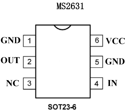
SOT23-6 封装图
