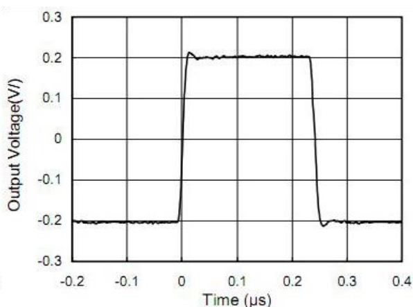
图 4. 小信号阶跃响应
