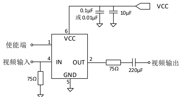
图 14. 直流耦合输入和交流耦合输出应用原理图
