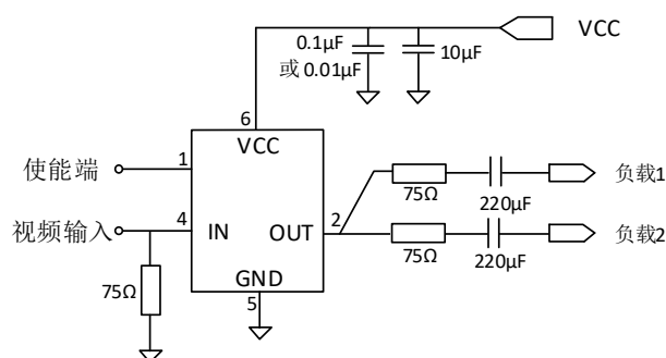
图 17. 机顶盒中直流耦合电路原理图
