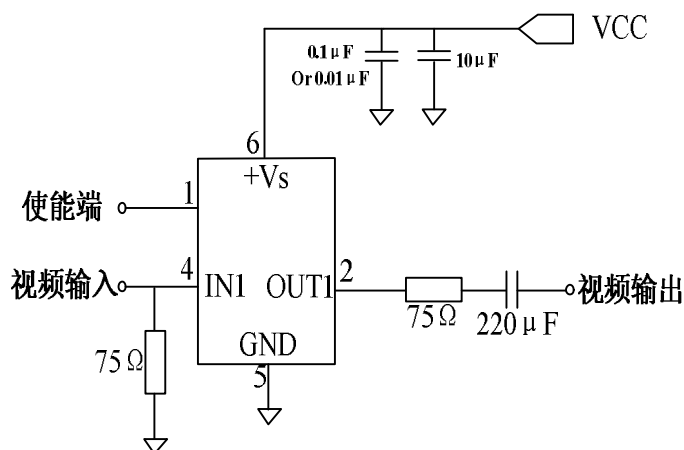
图 15. 直流耦合输入和交流耦合输出应用原理图
