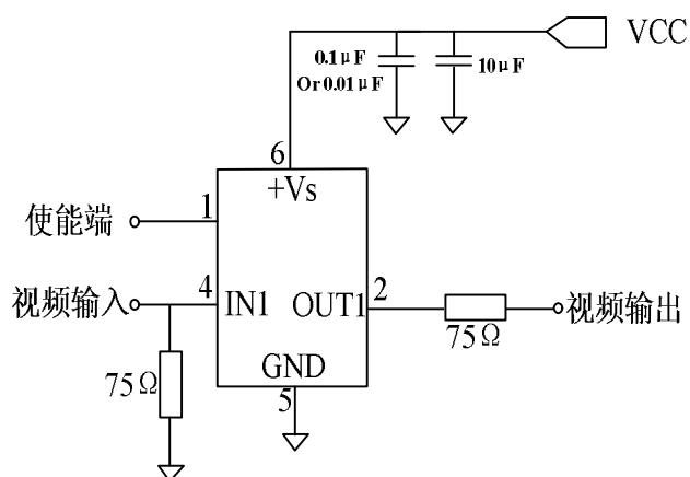
图 14. 直流耦合应用原理图
