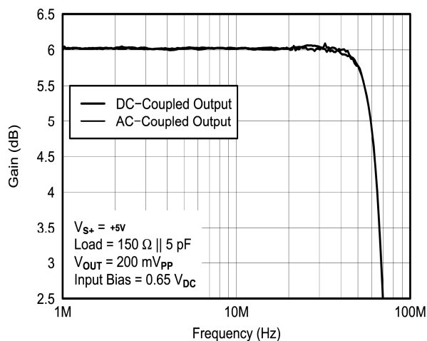
图 2. 频率响应
