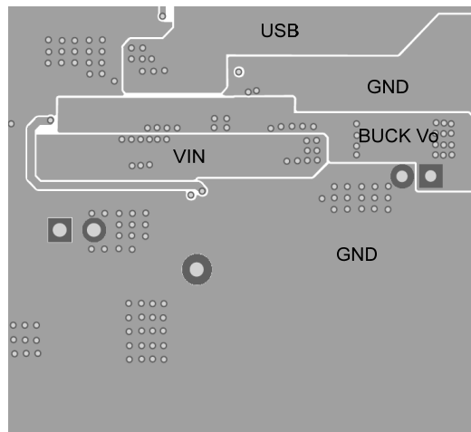
Bottom Layer
