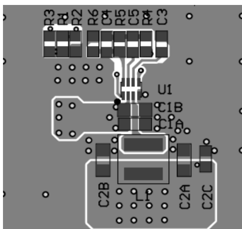
Top Layer
