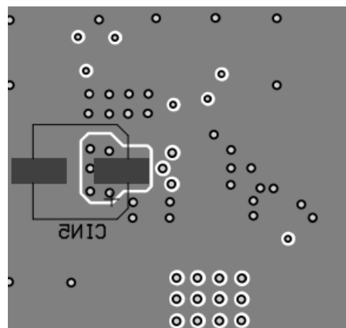
Bottom Layer
