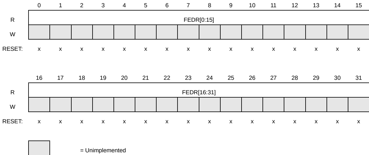
Figure 19-8. Flash ECC Data (FEDR) Register
