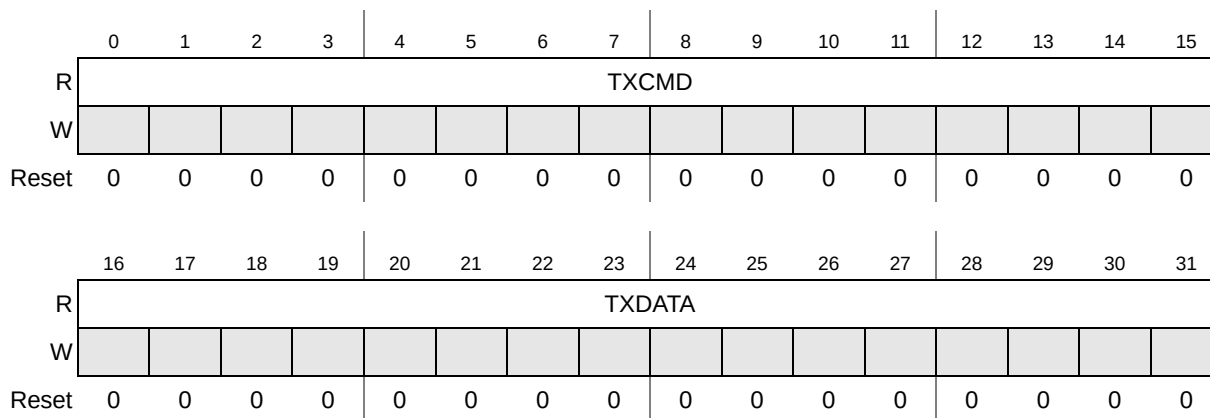
Figure 10-9. DSPI Transmit FIFO Register 0–4 (DSPIx_TXFRn)
