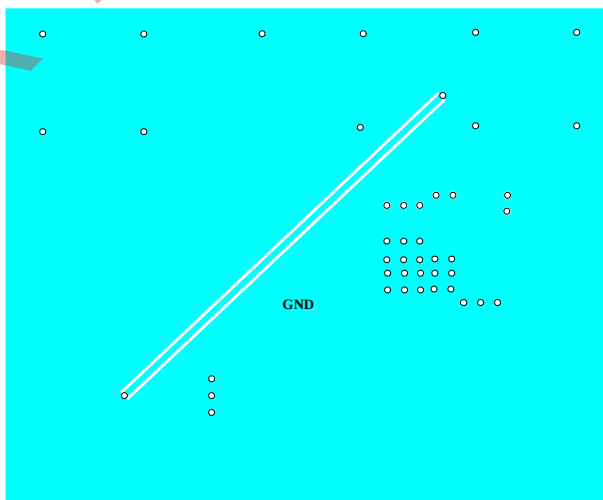
Inner2 Layer
