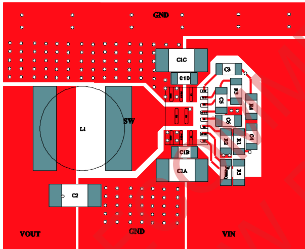
Top Layer
