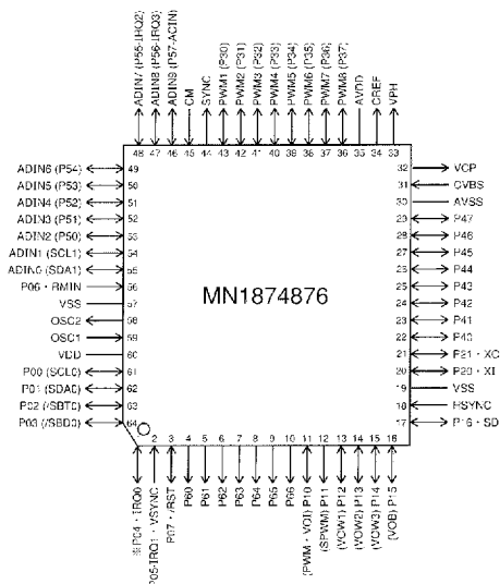
QFH064-P-1414B
