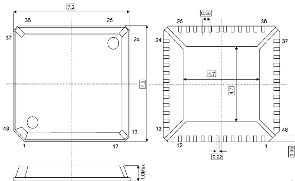
48 Pin VQFN
