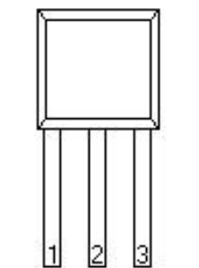
VSS VIN VOUT TO92 (Front View)
