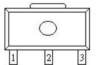
VSS VIN VOUT SOT-89 (Top View)
