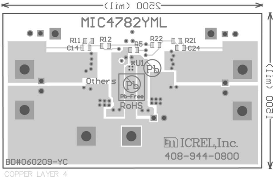
Bottom Layer
