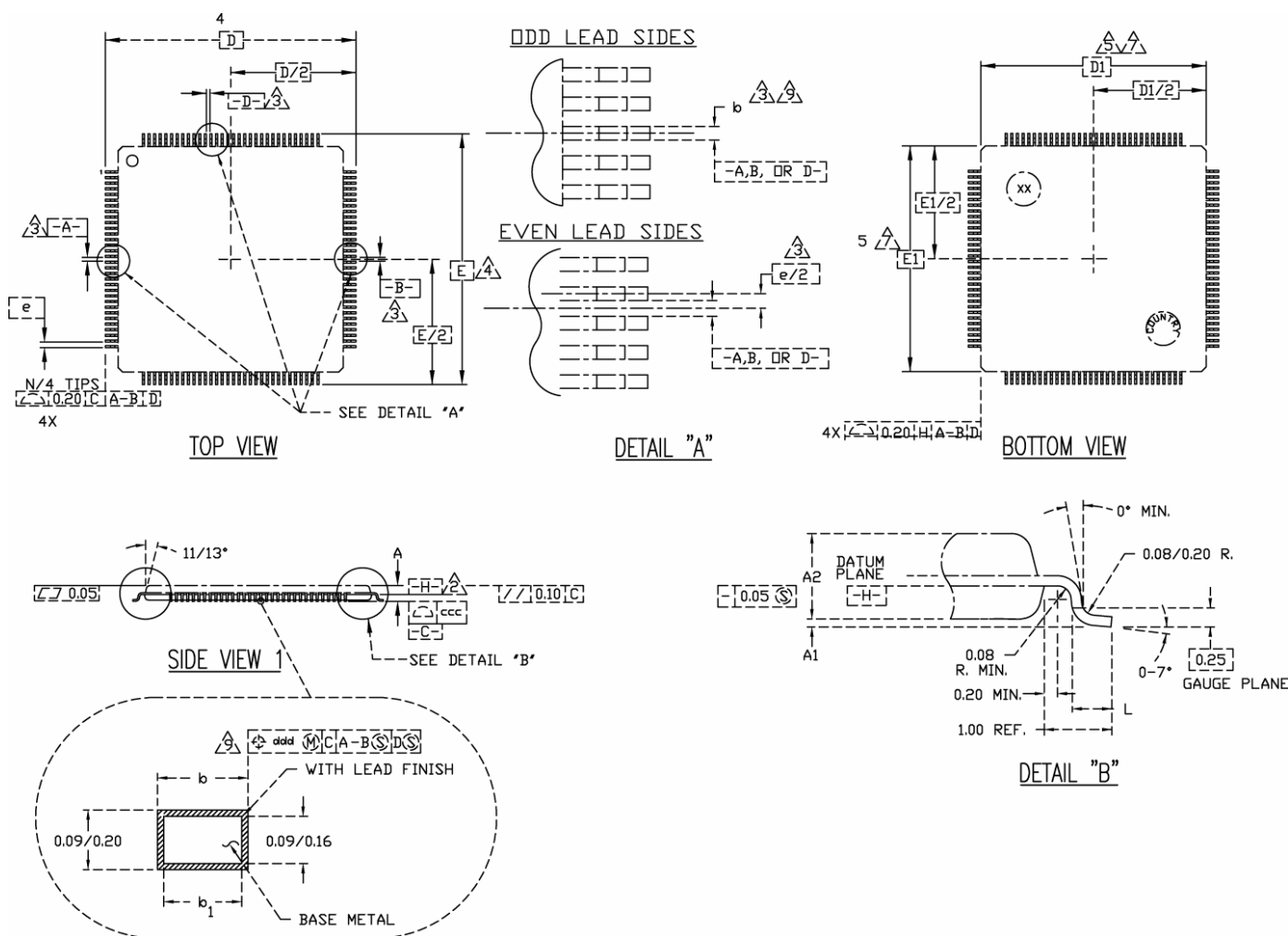
64-Pin (10x10x1.4) LQFP (V)
