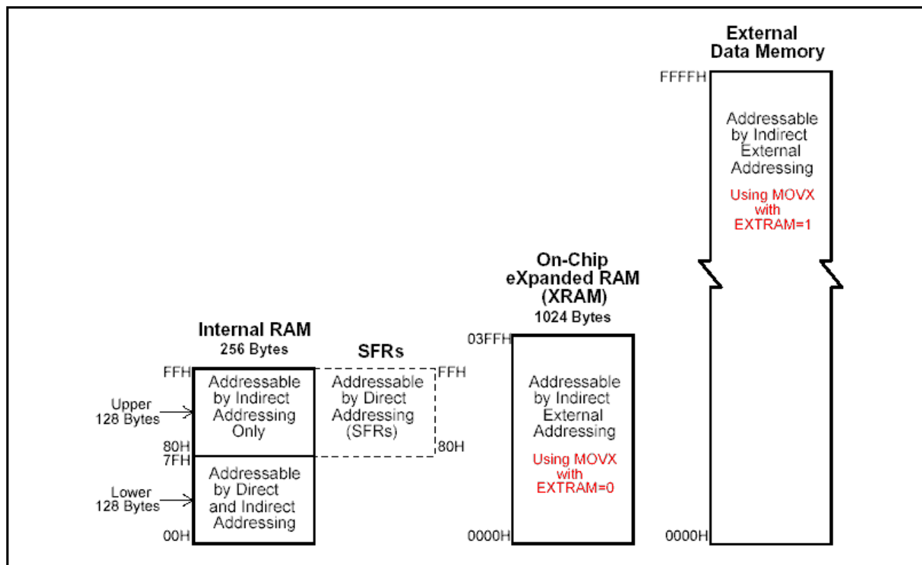
Figure 5-2. 数据存储器
