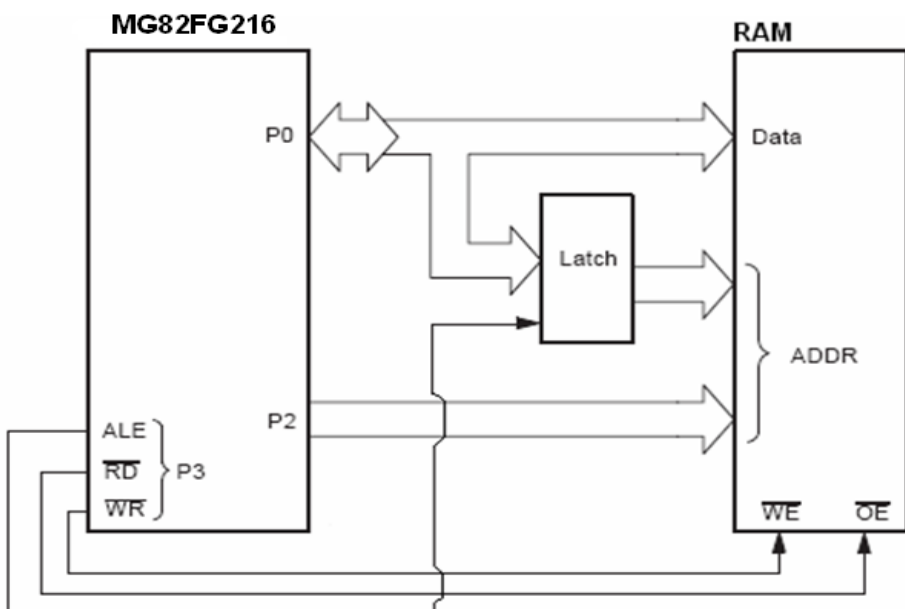
Figure 5-6. 通过16位地址访问外部RAM (使用 'MOVX @ DPTR')
