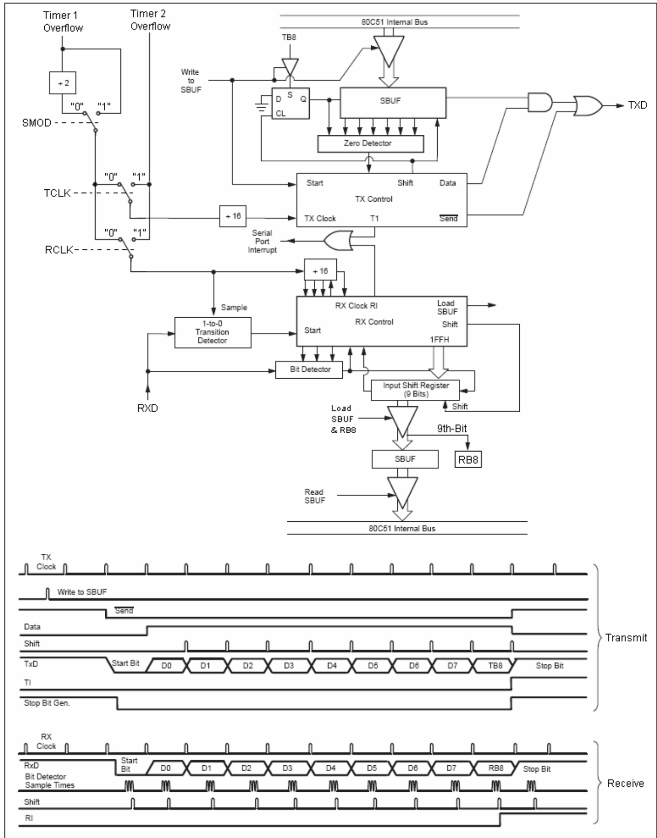
图 12-4 串行口模式 3
