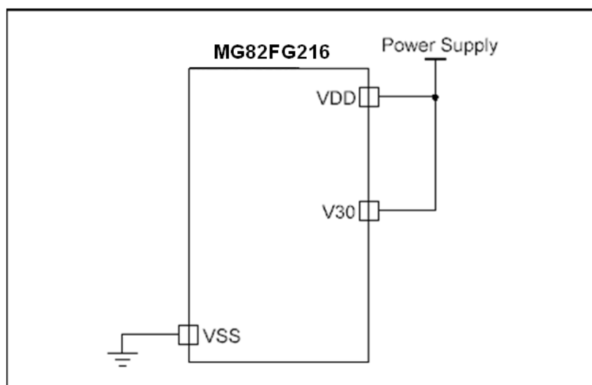
图27-2. 3.3V 供电
