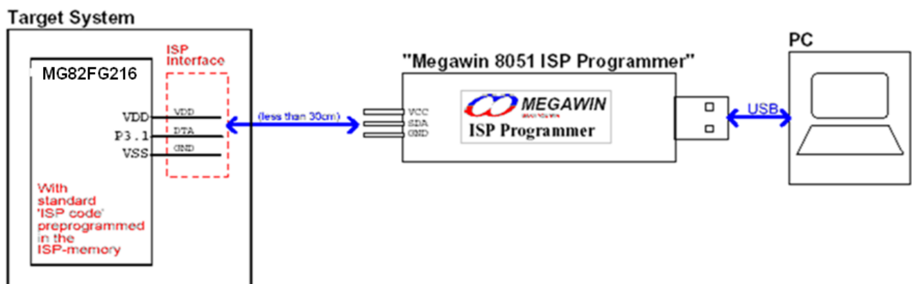
图 20-8. ISP 操作系统连接图
