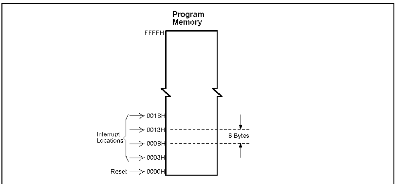
Figure 5-1. 程序存储器
