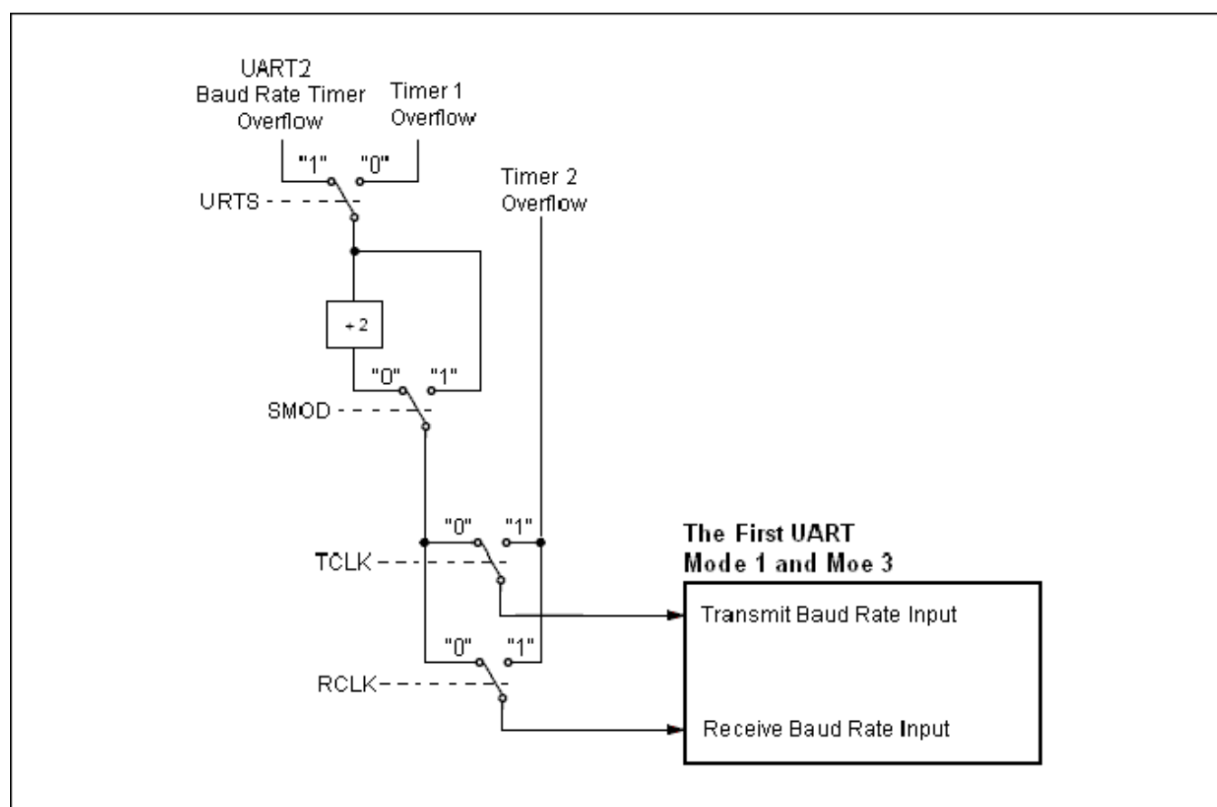
图 13-1. 标准UART的新波特率源
