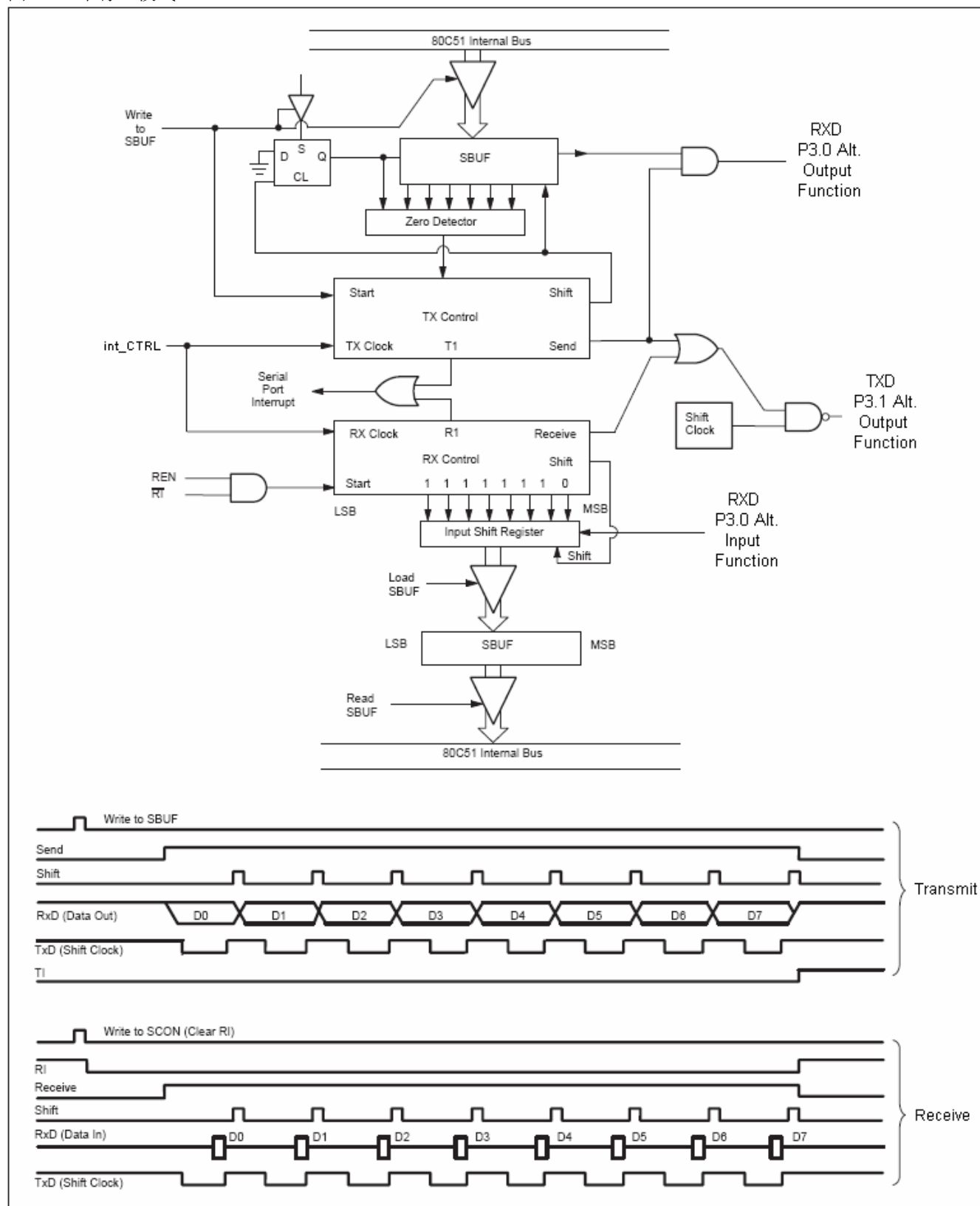
图 12-1 串行口模式 1
