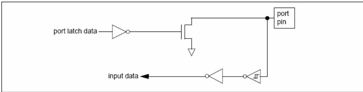
图 10-2 开漏输出
