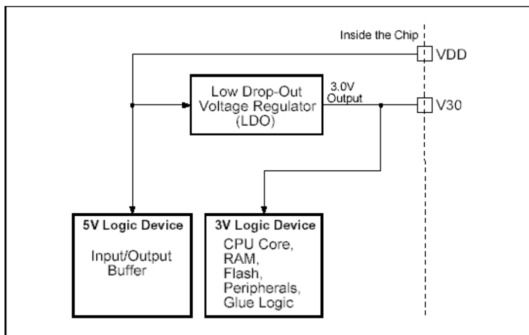
图 27-1. 电源电路
