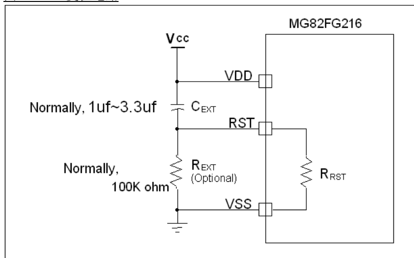
图 27-4. 复位电路
