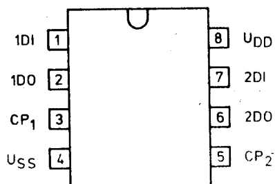
Układ wyprowadzeń
