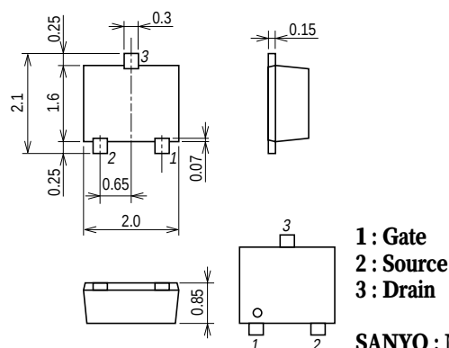
外形図 2167A
