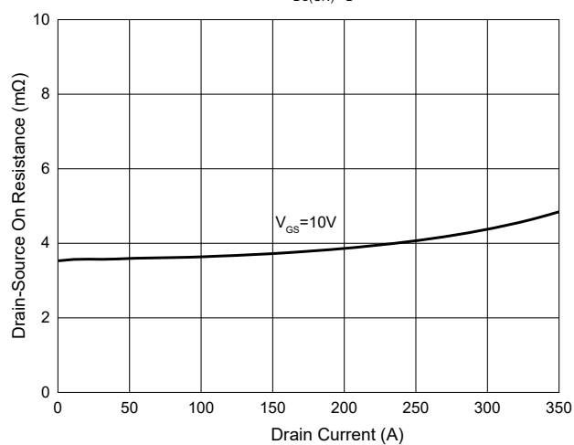
Fig. 4 - R_{DS(ON)} - I_D
