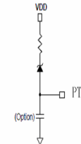
V_{DD} \text{ OVP : } V_{DD} > V_R + V_Z + 4V VDD OVP Only
