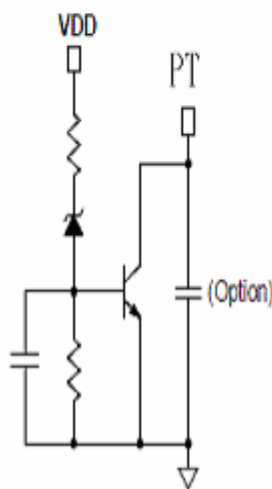
VDD OVP
