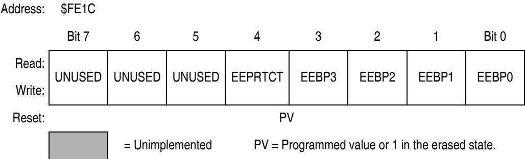
Figure 5-4. EEPROM-1 Nonvolatile Register (EE1NVR)
